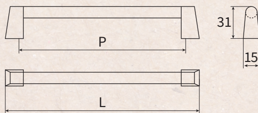
寸法図 (mm)
