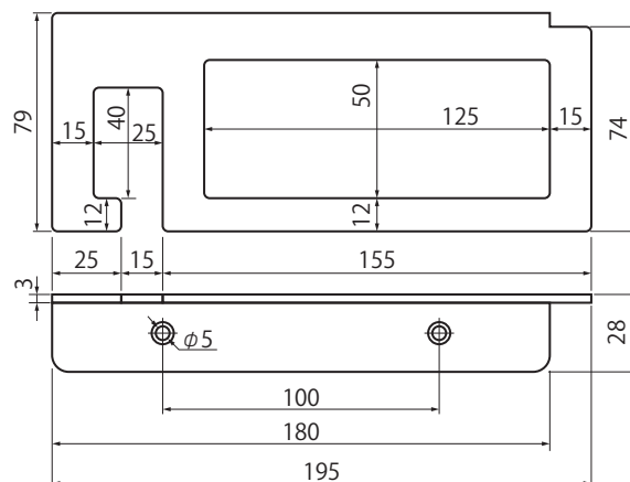
寸法図 (mm)
