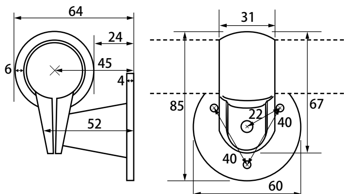
●寸法図 (mm)
