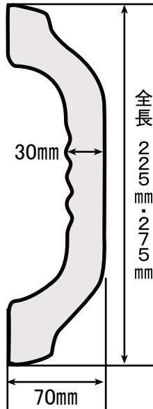
■寸法図
