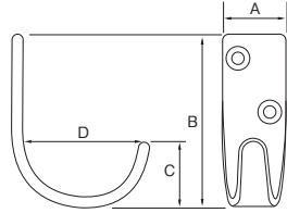
板厚 3t
