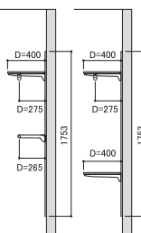
A断面図 B断面図
