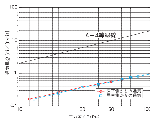
気密等級線グラフ
