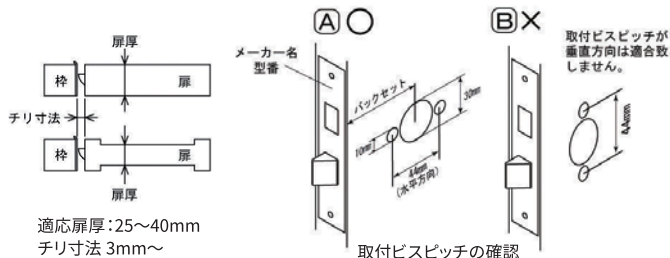
取付ビスピッチの確認
