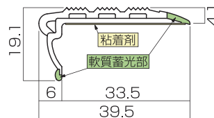
製品断面 (mm)
