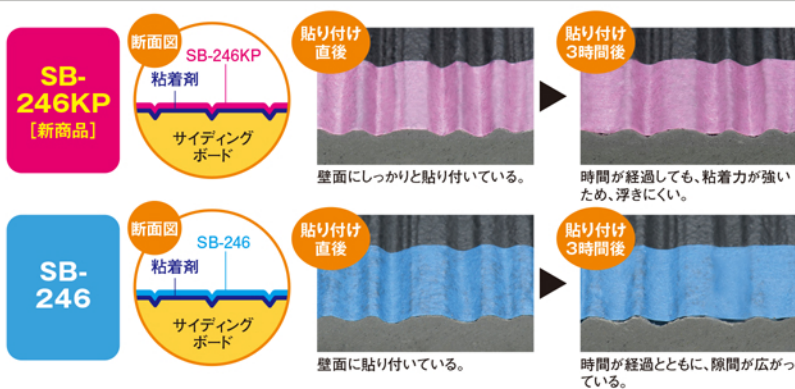
「SB-246KP」のサイディングボード貼り付け比較試験
