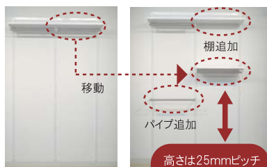
※当社 公的試験時写真 (100kg 負荷時)
