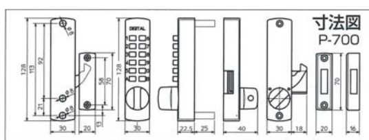
P-700 (引戸兼用面付錠固定サムターン)
