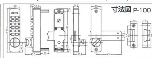
寸法図 P-700
