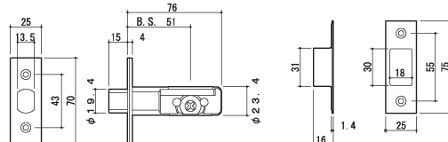
●専用ラッチ寸法図
