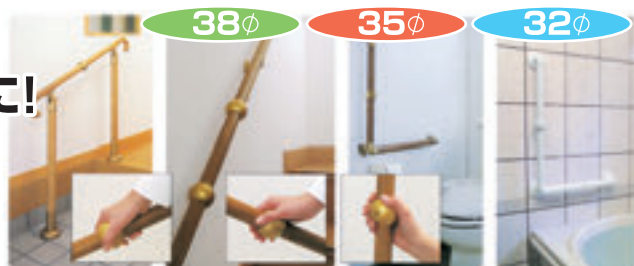
BR-64 どこでもグリップボール形 (亜鉛合金/ナベ4X16)
