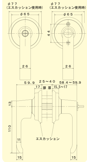
<寸法図>
