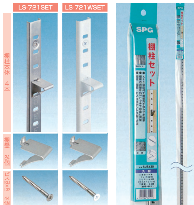
棚柱本体:形状図
