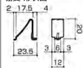
棚受:形状図
