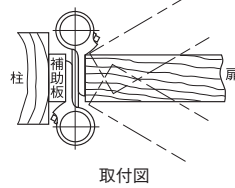
取付図
