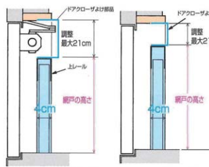
ドアクローザをよける取付け例 ※ドアクローザがない場合でも高さ調整に利用します。
