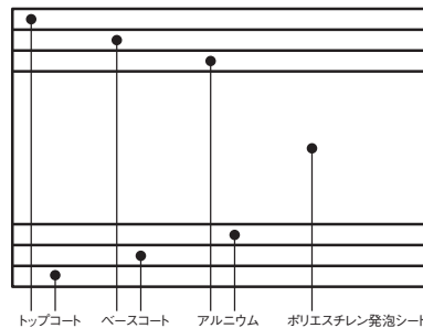
両面塗装品 断面構成図
