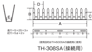
TH-308SA (継続用)
