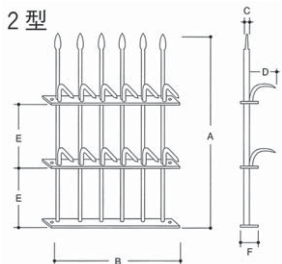
忍び返し2型
