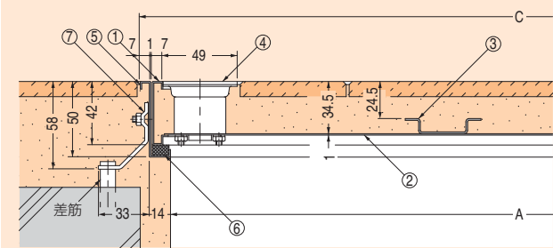
モルタル充填用(充填深さ:24.5mm) 樹脂タイル貼物用(適用床材:4mm以下)
