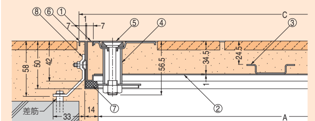
モルタル充填用(充填深さ:24.5mm) 樹脂タイル貼物用(適用床材:4mm以下)
