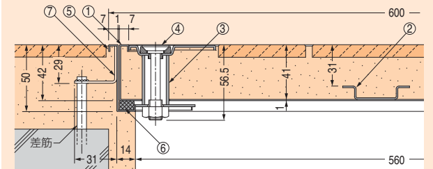
モルタル充填用(充填深さ:31mm)
