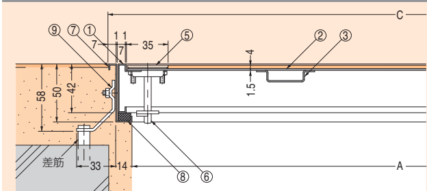
樹脂タイル貼物用
