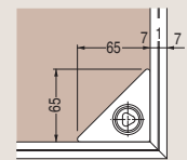
ロック部 平面詳細
