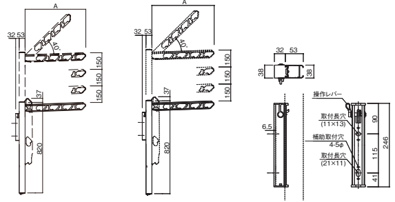
■取付ブラケット詳細図
