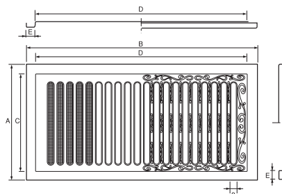
UK-YK 2040-BKM
