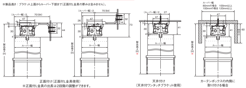
■側面図
