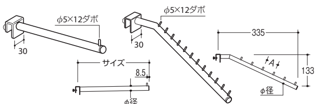
Vフェイスアウトハンガー
