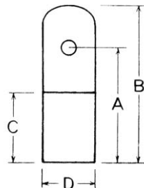
※丸パイプの肉厚は0.8mm
