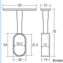
ブラケット エンド
