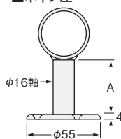
■木ネジ座
