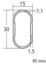
アルミハンガーパイプ 500mm/1000mm/2000mm
