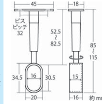
アジャストブラケット エンド (伸縮タイプ)
