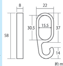
フック ホワイト (耐荷重3kg)
