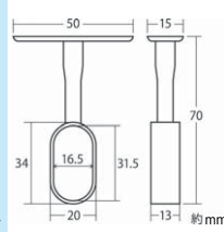
ブラケット バス
