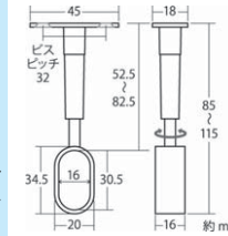
アジャストブラケット バス (伸縮タイプ)
