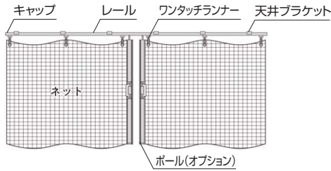
【ネット・メッシュカーテン】構成図
