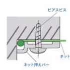
天井・壁面取付
