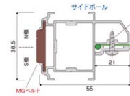
間仕切サイドポール【押えバタイプ】取付
