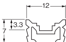
掘込み寸法 12 × 7
