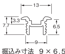
掘込み寸法 9 × 6.5
