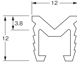
掘込み寸法 12×12
