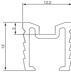
掘込み寸法 12×12
