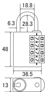
●寸法図(mm)
