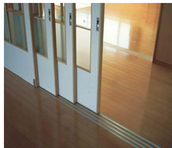
掘込み寸法 9×9 ( )の数字は12タイプ 12×12
