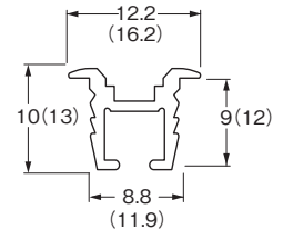
掘込み寸法 9×9 ( )の数字は12タイプ 12×12
